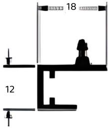
MONTANTE MÃO DE AMIGO COM REFORÇO
