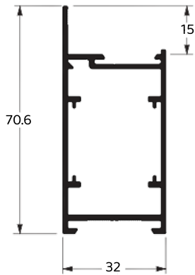
MONTANTE PARA PORTA DE GIRO
