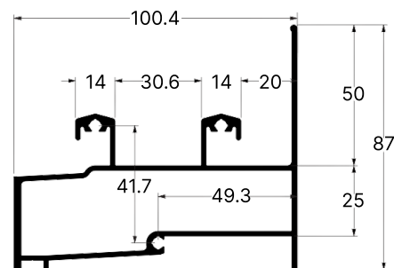
TRILHO COLUNA
