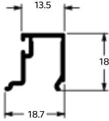
BAGUETE
