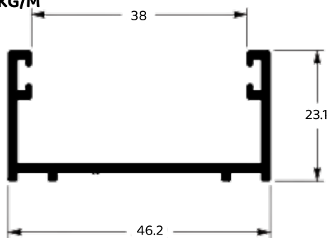
BAGUETE EM U - MATA JUNTA
