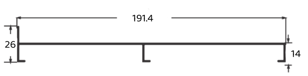
MARCO LATERAL LISO 04 FOLHAS
