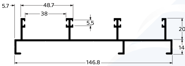
LATERAL 03 FOLHAS
