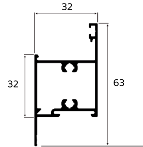
TRAVESSA MAXIM AR FIXO
