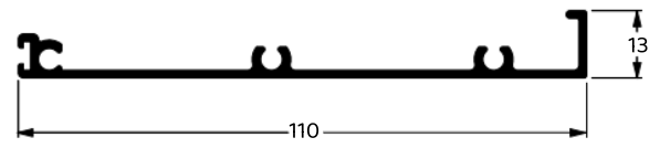
MARCO INTERMEDIÁRIO DA INTEGRADA
