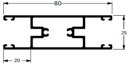
GUIA DUPLA DA PERSIANA INTEGRADA
