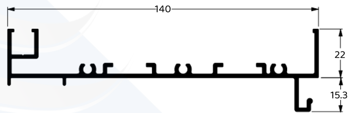
MARCO SUPERIOR DA CAIXA DA PERSIANA
