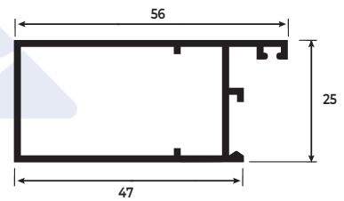
MONTANTE PARA PORTA
