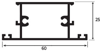
TRAVESSA PARA PORTA
