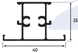
TRAVESSA PARA PORTA
