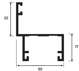
MARCO PARA MAXIM AR
