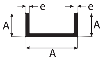
Perfil U com abas e bases desiguais
