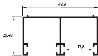
TRILHO SUPERIOR DUPLO
