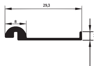
TRILHO INFERIOR
