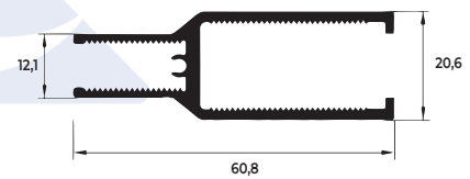
LEITO PARA 8MM
