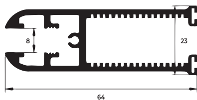
LEITO PARA 8MM
