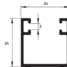
TRILHO SUPERIOR SIMPLES
