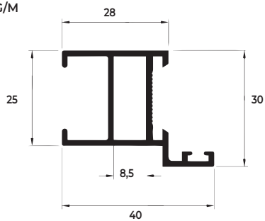
PORTAL BATENTE
