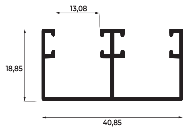
BX-5898 0,320 KG/M
