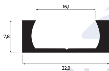
TRILHO INFERIOR
