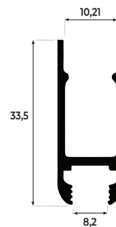
BX-6000 0,304 KG/M
