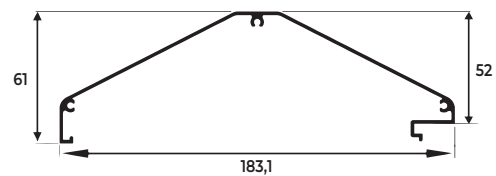
TAMPA INTEGRADA
