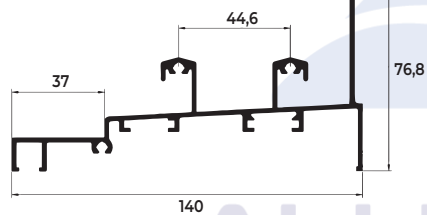
MARCO INFERIOR
