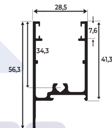
TRAVESSA DA FOLHA
