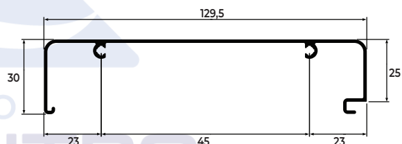
TAMPA INTERNA JANELA INTEGRADA
