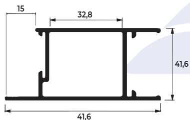
LG-050 0,816 KG/M
