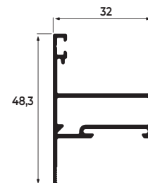
MONTANTE DA FOLHA MAXIM AR
