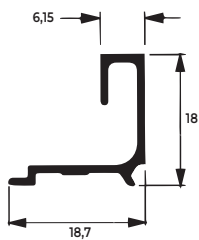
BAGUETE PARA VENEZIANA VZ-006
