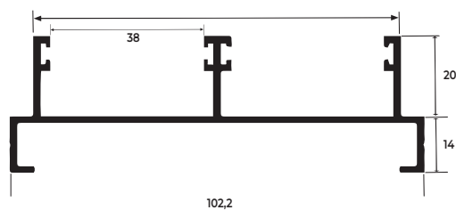
MARCO LATEREAL 02 FOLHAS
