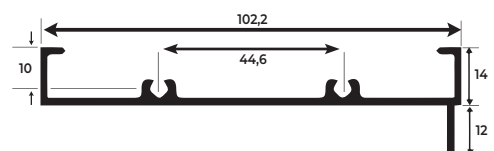
MARCO LATEREAL COM FRESA
