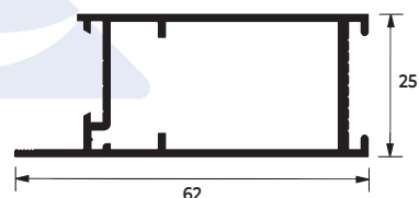
SU-111 0,614 KG/M
