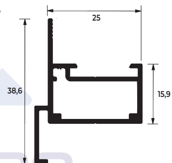
TRAVESSA / FOLHA
