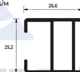
TRAVESSA SUPERIOR DA FOLHA MAXIM AR
