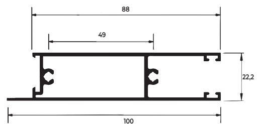
SU-225 0,983 KG/M
