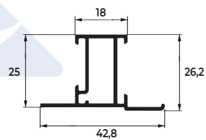
MONTANTE FOLHA
