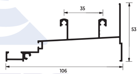
SU-025 0,919 KG/M
