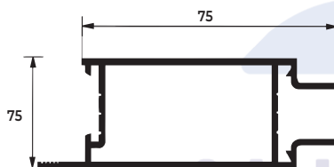
SU-244 0,682 KG/M
