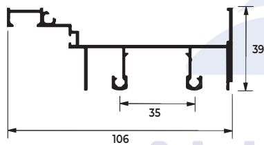
MARCO SUPERIOR CORRER JANELA CAMARÃO
