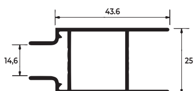
SU-191 0,683 KG/M
