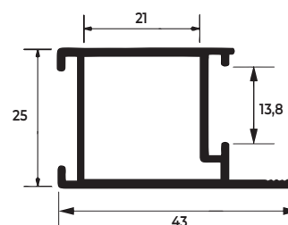
MONTANTE DA FOLHA
