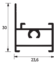
TRAVESSA PA FOLHA COM OLHAL
