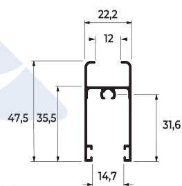
TRAVESSA DA FOLHA VENEZIANA
