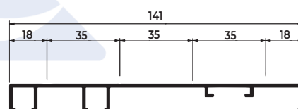
SU-123 0,857 KG/M
