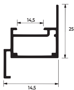
SU-098 0,401 KG/M
