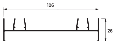
SU-013 0,738 KG/M
