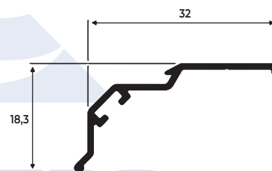
SU-083 0,144 KG/M
