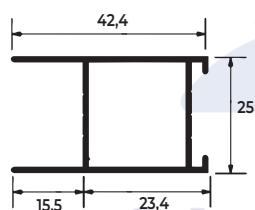
MONTANTE / FOLHA VENEZIANA
