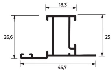
SU-200 0,418 KG/M
