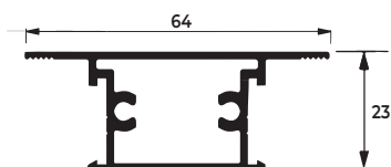
SU-227 0,540 KG/M
