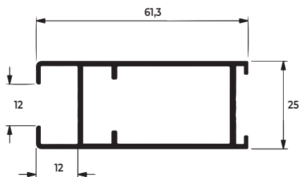
SU-241 0,668 KG/M
