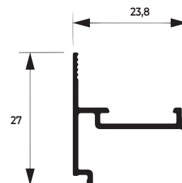
PERFIL REVERSOR
