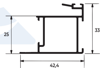
SU-041 0,485 KG/M
