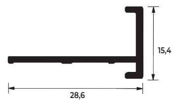
MATAJUNTA
