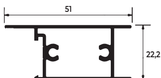
TRAVESSA / FOLHA
