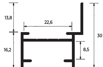
MONTANTE CENTRAL
