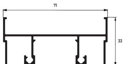
SU-001 0,738 KG/M
