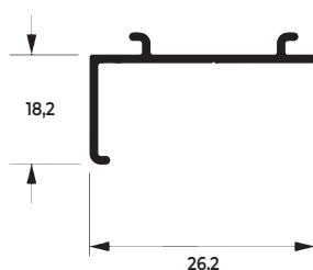
PINGADEIRA FOLHA
