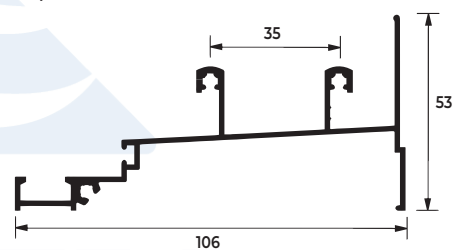
SU-025 0,919 KG/M
