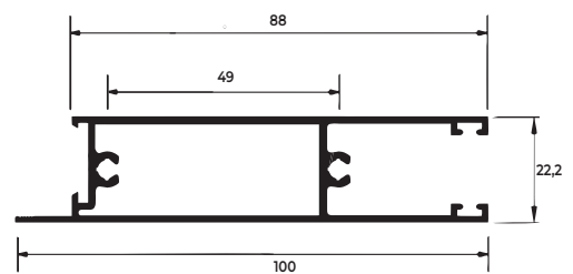
SU-225 0,983 KG/M
