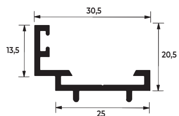
COMPLEMENTO / FOLHA
