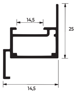
SU-098 0,401 KG/M
