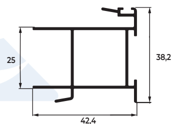
SU-069 0,600 KG/M
