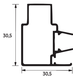
VEDAÇÃO MONTANTE
