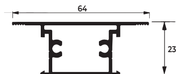
SU-227 0,540 KG/M
