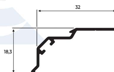
SU-083 0,144 KG/M
