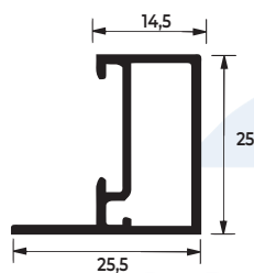
MONTANTE / FOLHA
