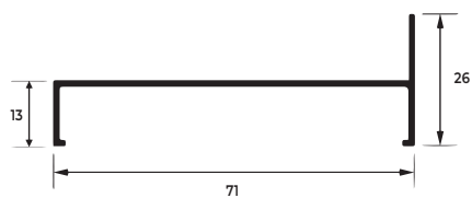
SU-007 0,371 KG/M
