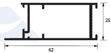
SU-111 0,614 KG/M
