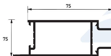
SU-244 0,682 KG/M
