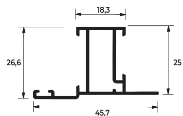
SU-200 0,418 KG/M
