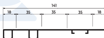
SU-123 0,857 KG/M
