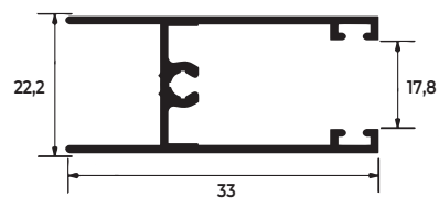
TRAVESSA FOLHA
