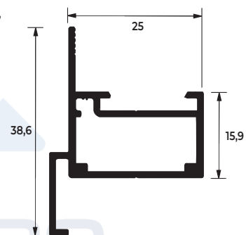
TRAVESSA / FOLHA
