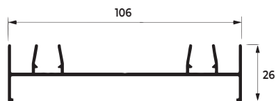
SU-013 0,738 KG/M
