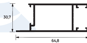
SU-245 0,676 KG/M
