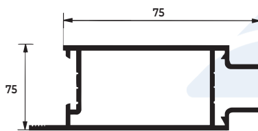
SU-244 0,682 KG/M
