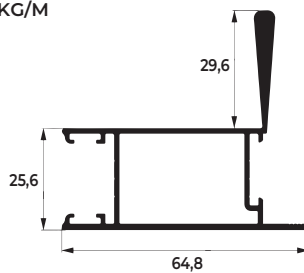
MONTANTE LATERAL FOLHA
