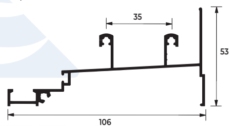
SU-025 0,919 KG/M
