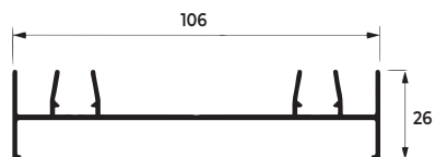
SU-013 0,738 KG/M
