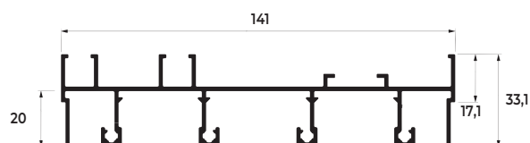
MARCO SUPERIOR DE CORRER 4 FOLHAS
