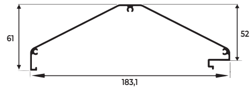
TAMPA INTEGRADA
