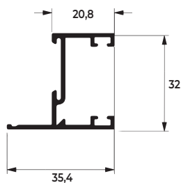
MARCO LATERAL MAXIM AR
