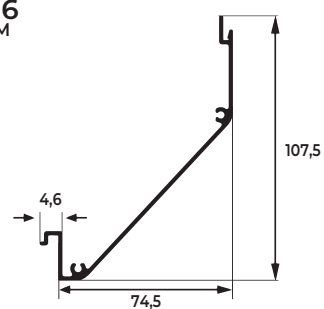
TAMPA INTERNA INFERIOR DA CAIXA INTEGRADA
