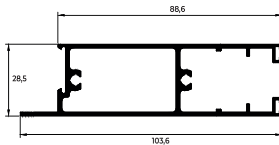
TRAVESSA INFERIOR COM ESCOVINHA
