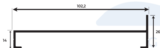
MARCO LATEREAL LISO 02 FOLHAS
