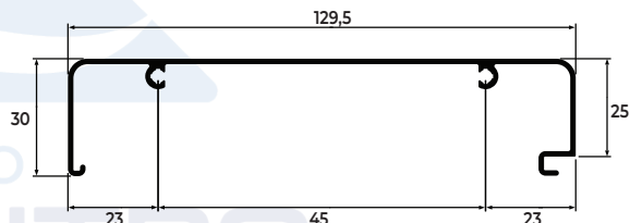
TAMPA INTERNA JANELA INTEGRADA
