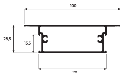
TRAVESSA LARGA DA FOLHA
