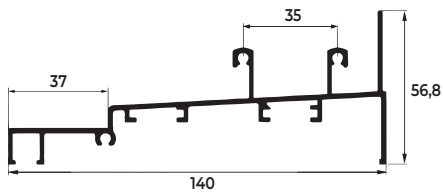
TRILHO INFERIOR
