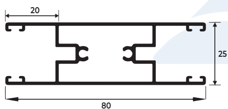
MN-027 1,043 KG/M
