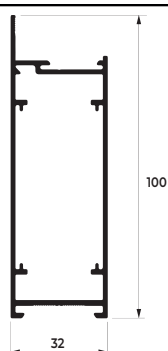
MONTANTE DA FOLHA - PORTA DE GIRO
