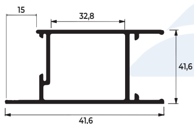
LG-050 0,816 KG/M
