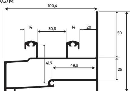
TRILHO COLUNA
