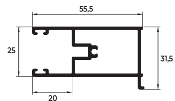
MN-007 0,710 KG/M
