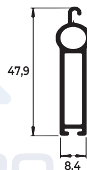
TERMINAL DA PERSIANA BRUTO
