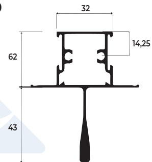
MONTANTE MAXIM AIR
