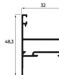
MONTANTE DA FOLHA MAXIM AR
