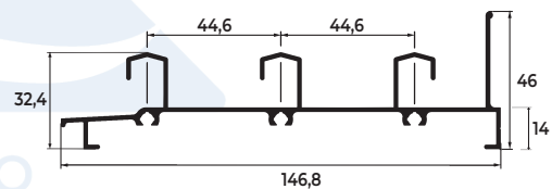
TRILHO INFERIOR 03 FOLHAS
