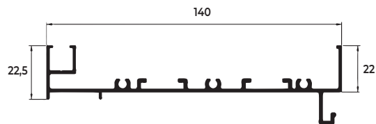
MN-001 1,377 KG/M
