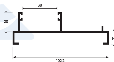
LG-124 0,773 KG/M
