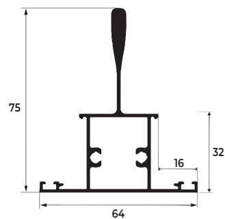
MONTANTE MAXIM AR
