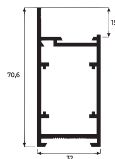
MONTANTE PARA PORTA DE GIRO
