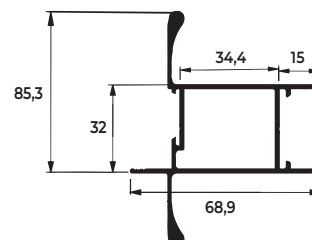
LG-201 1,195 KG/M
