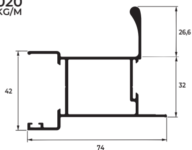
MONTANTE LATERAL COM ABA E PUXADOR INTERNO
