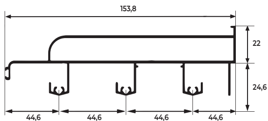
PERFIL PARA LINHA GOLD
