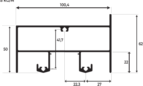
TRAVESSA BANDEIRA PORTA/JANELA
