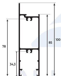
TRAVESSA INFERIOR DA FOLHA
