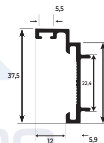
COMPLEMENTO DA FOLHA BATENTE
