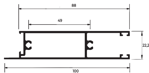
SU-225 0,983 KG/M
