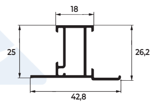
MONTANTE FOLHA
