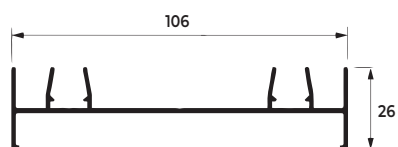
SU-013 0,738 KG/M
