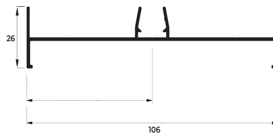
SU-014 0,639 KG/M
