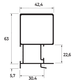
MONTANTE MÃO DE AMIGO TUBULAR SEM ESCOVINHA
