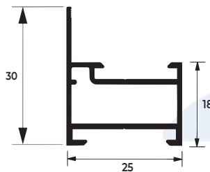
TRAVESSA SUPERIOR FOLHA
