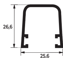
VEDAÇÃO MONTANTE
