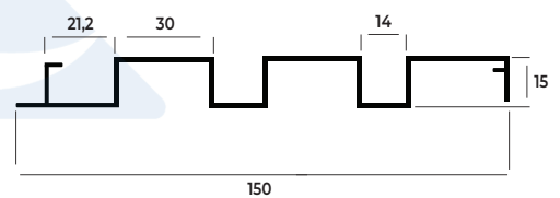
DP-073 0,771 KG/M
