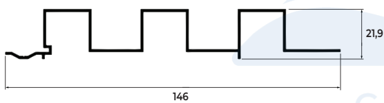
DP-074/L 0,859 KG/M
