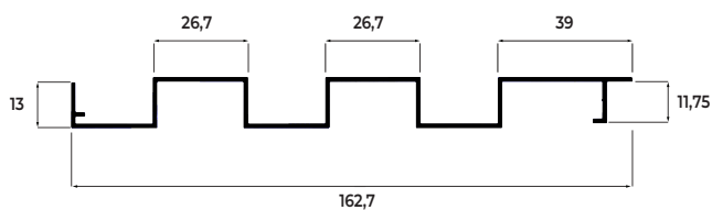
DP-075 0,907 KG/M
